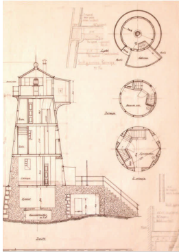
Snitttegning
